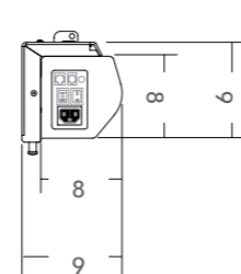
Côté du carter avec patte de fixation Side of the case with bracket
